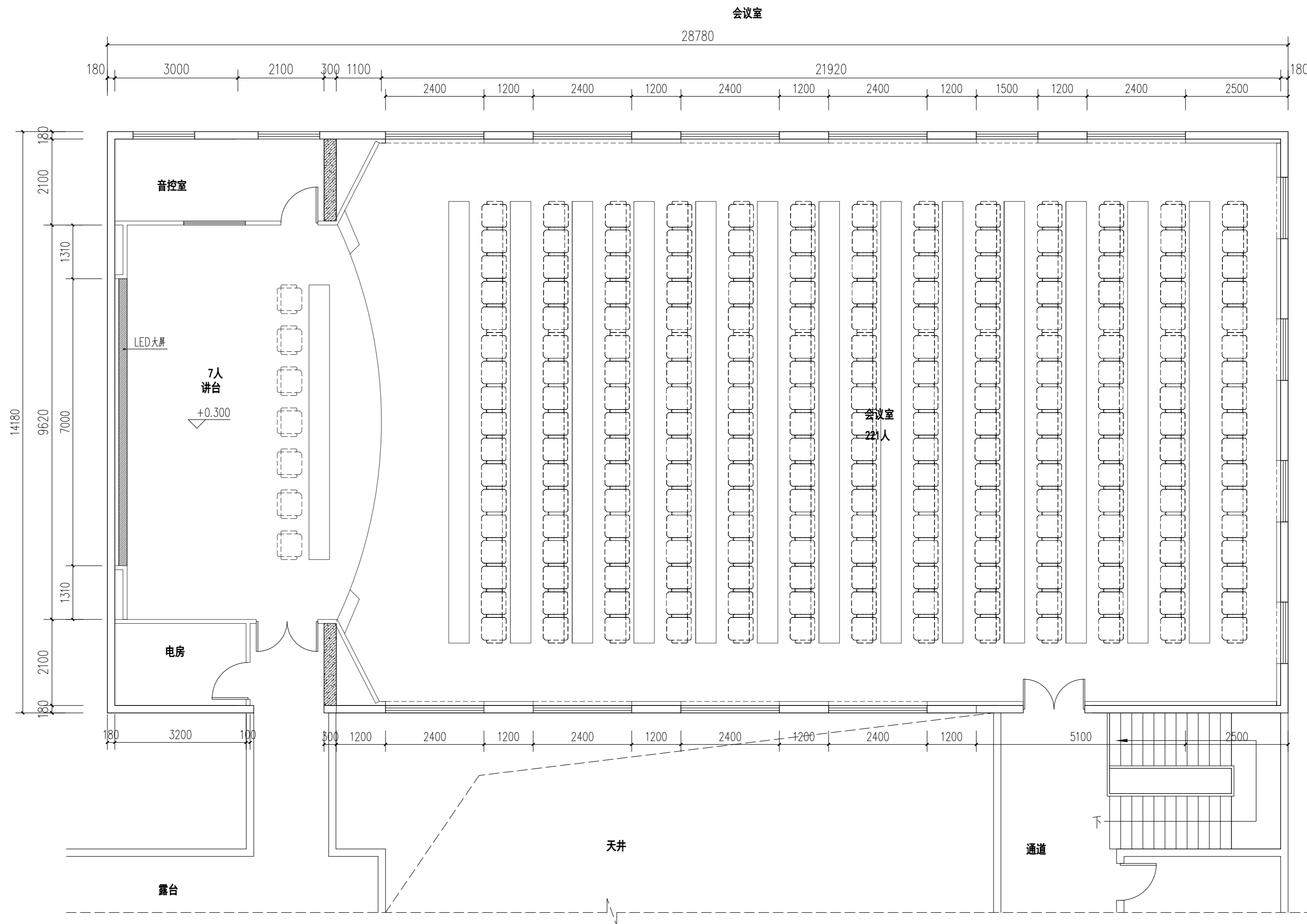
会议室升级改造平面布置图 1:80
