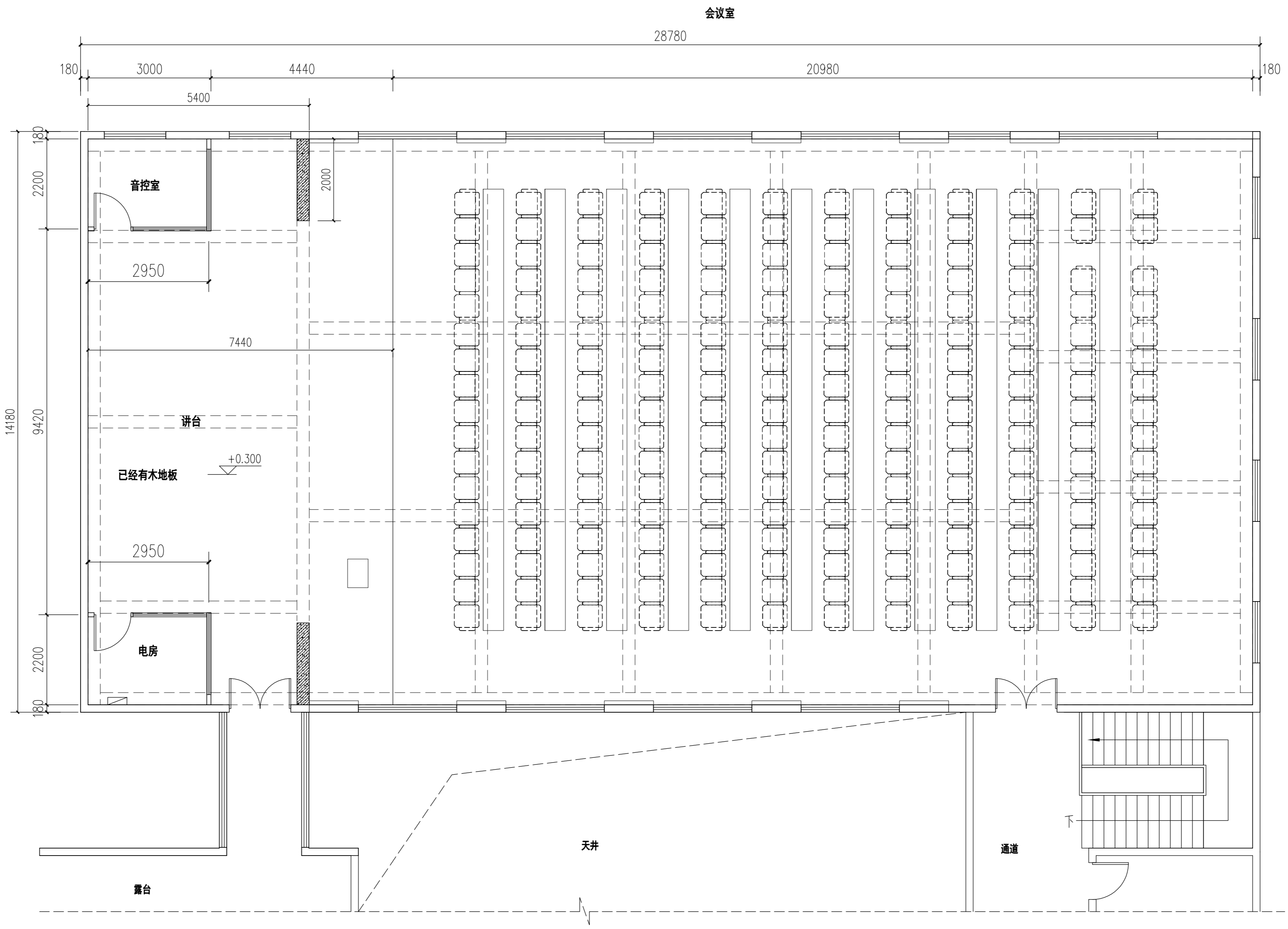
会议室现场平面布置图 1:80
